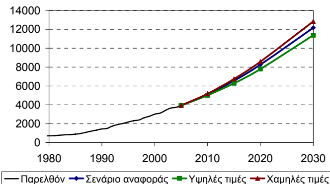
Τελική κατανάλωση ηλεκτρισμού (GWh)
